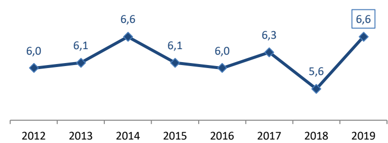
Gráfico 6. Caudal (m3/s) tratado por la PTAR-C en Cali (2012 – 2019)
